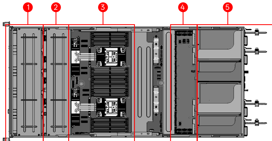
图5-4 内部视图-CPU层
