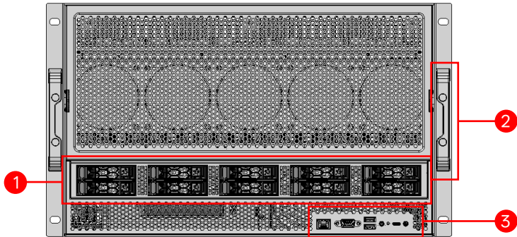
图3-1 前面板视图
