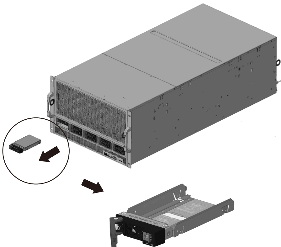
图5-4 卸下硬盘托架
