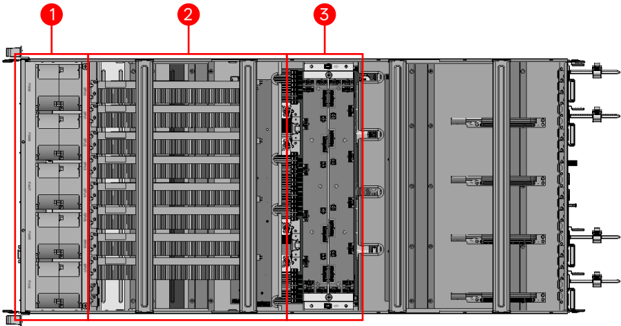
图3-4 内部视图-GPU层
