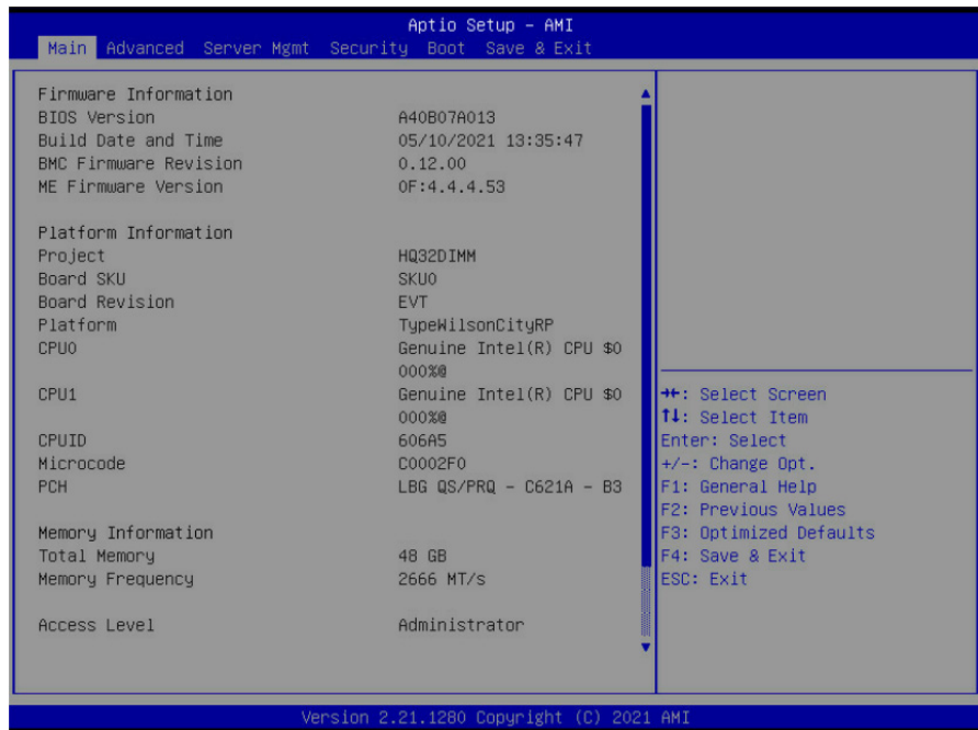
图8-4-1 Main界面
