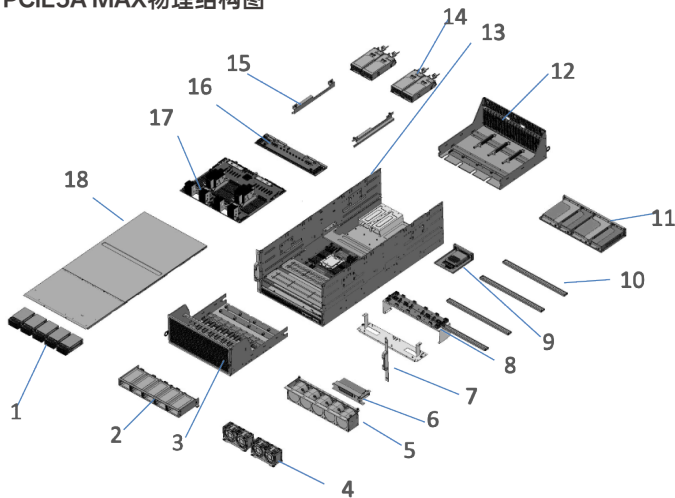
图4 G5208 PCIe5A MAX物理结构图
