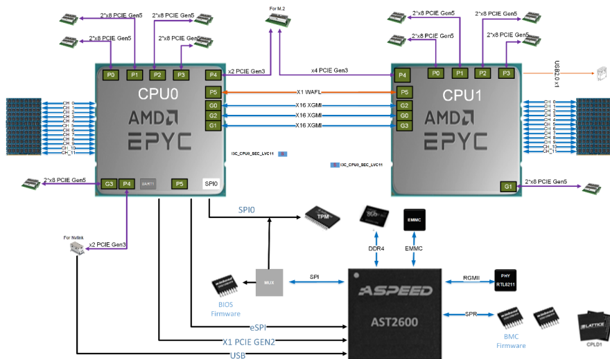
图3 G5208 PCIE5A MAX主板逻辑架构图
